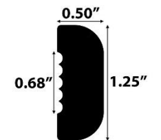
Mini Adjustable Stair Nose WPC (059)
