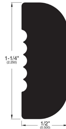
STAIR NOSE MINI ADJUSTABLE WPC (059)
